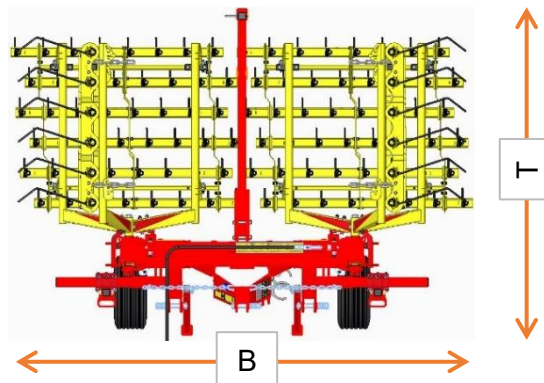
Abbildung 16: AS - Ansicht von oben in Transportstellung
