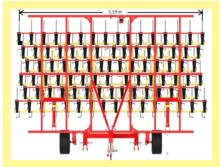
Abbildung 21: Striegelfeldbreite VS 300 M1
