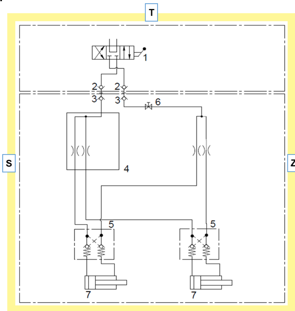
Abbildung 25: Hydraulikschemata VS 300 M1
