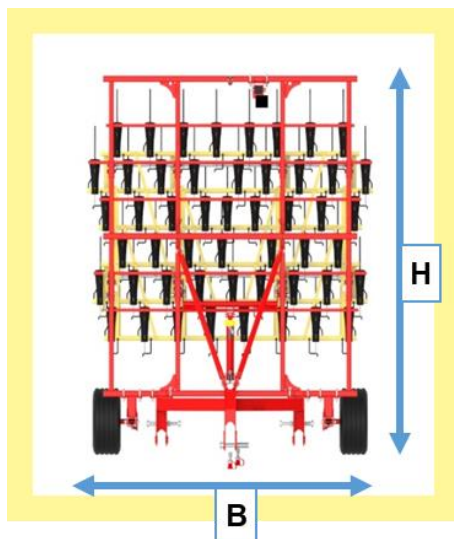
Afbeelding 22: vario-cultuureg - bovenaanzicht in transportstand
