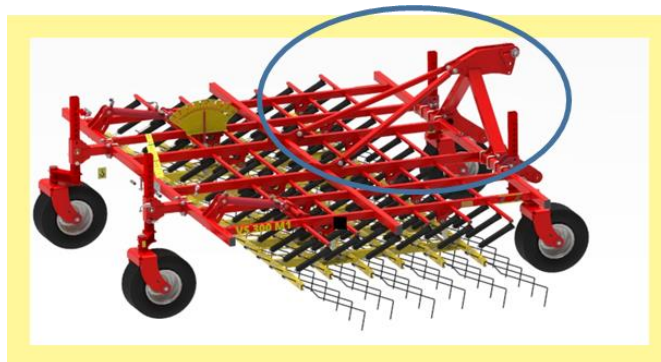
Afbeelding 14: montage van de aanbouwbok en de trekstangen
