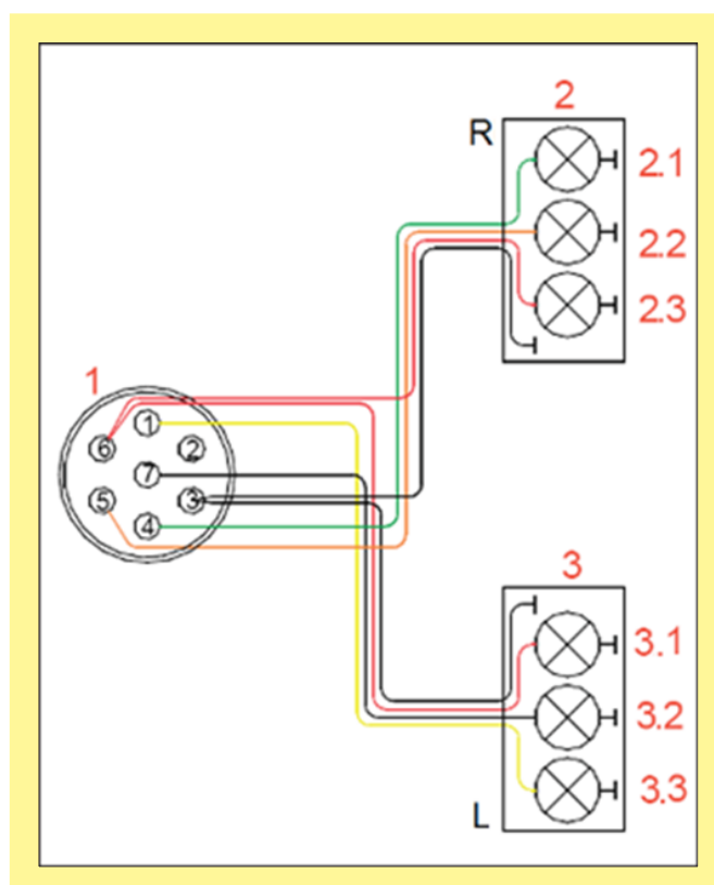
Afbeelding 27: schakelschema
