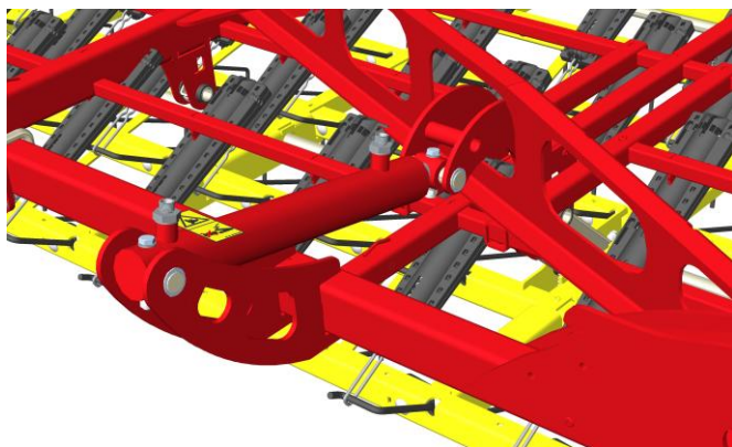
Abbildung 13: Hydraulikzylinder
