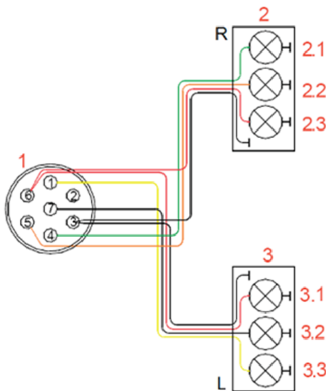
Abbildung 37: Schaltbild
